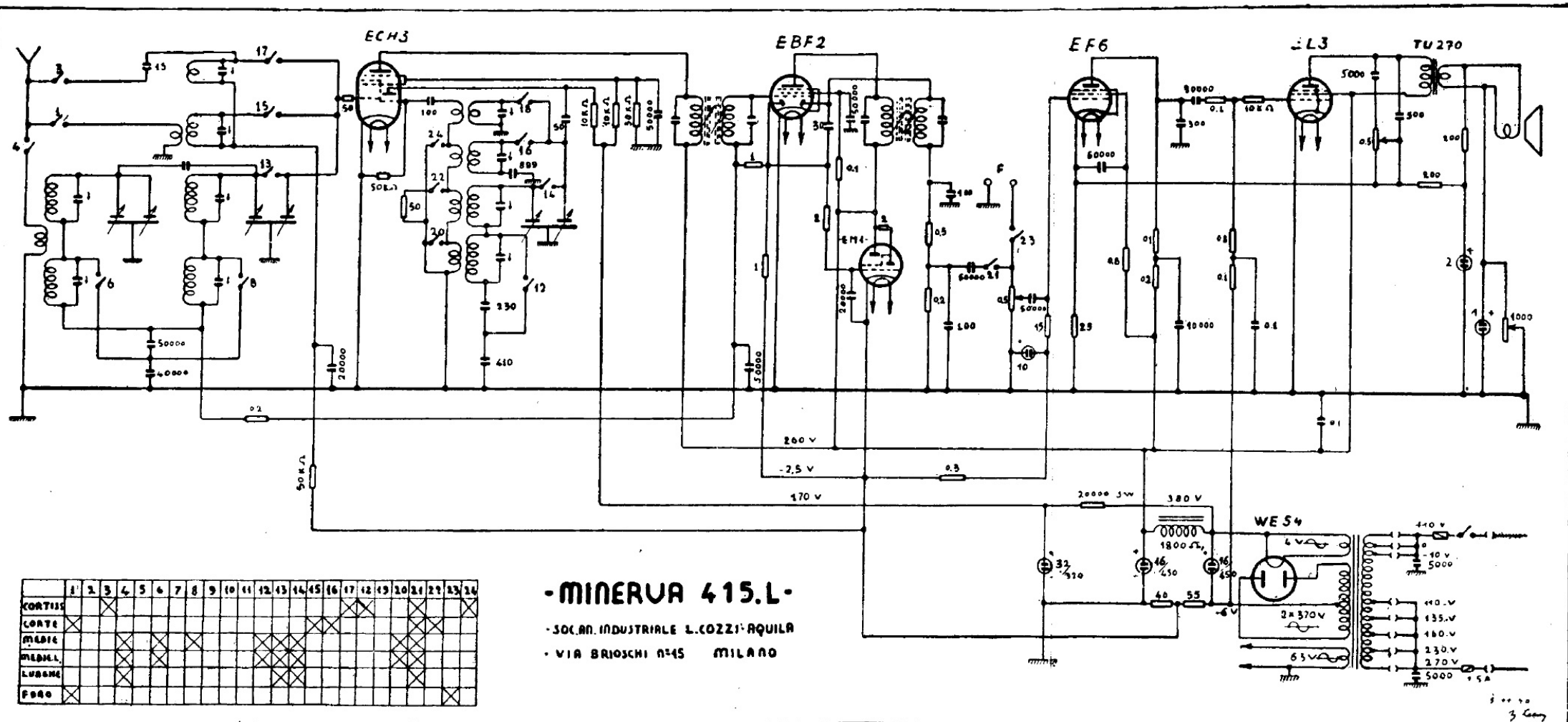
MINERVA RADIO. — Mod. « 415 L » e « 1415 ». — Gamme: lunghe, da 300 a 2000 m., medie da 190 a 580 m., corte da 26 a 52 m., cortissime da 13 a 26 m. — Produzione 1940-1941. — Media frequenza: 470 kHz. (Stesso schema anche per i modd. « 406, 416 e 1416 », con stadio alta frequenza e valvola EF8).
